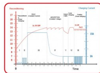
Διάγραμμα σταδίων φόρτισης / Diagram of charging stages
